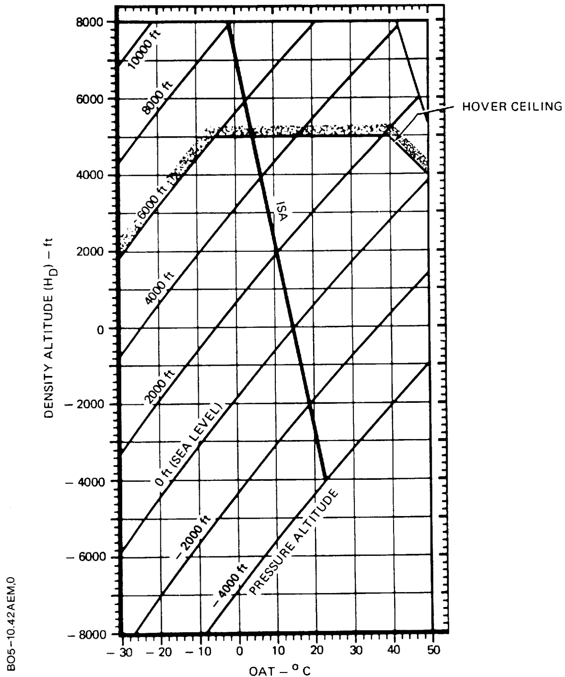
Fig. 3 Hover Ceiling I G E - GM 2400-2500 kg
